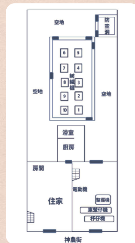
錦源興織布工廠機械配置圖(國家發展委員會檔案管理局的典藏文件的重繪圖)
